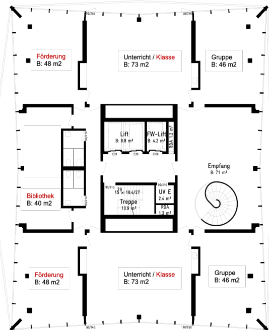
1. Obergeschoss, Raumhöhe: 3.14m (OKFB - UKD)
